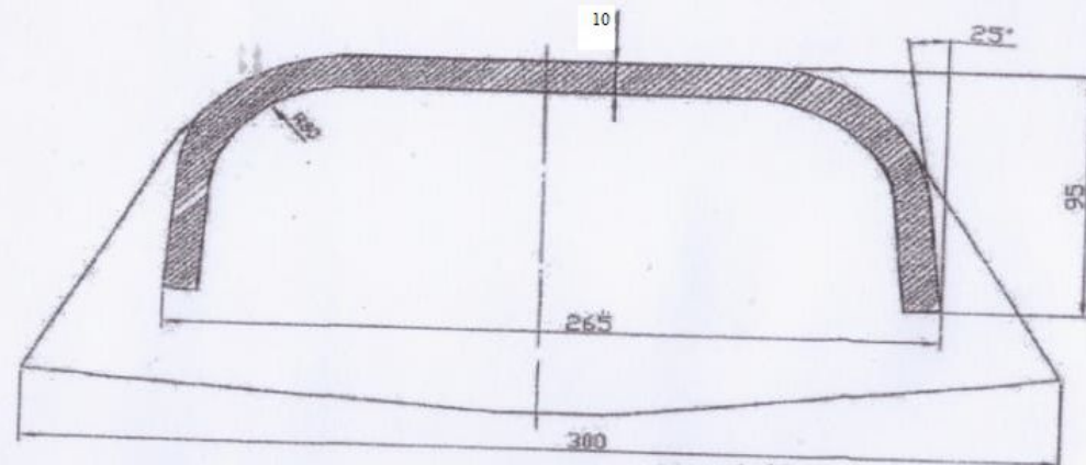
A-B Kesidi Section
